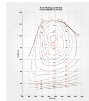
发动机油耗曲线
