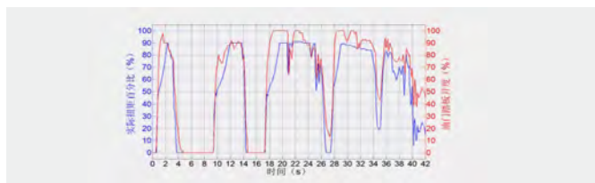
整车与底盘动力匹配曲线
